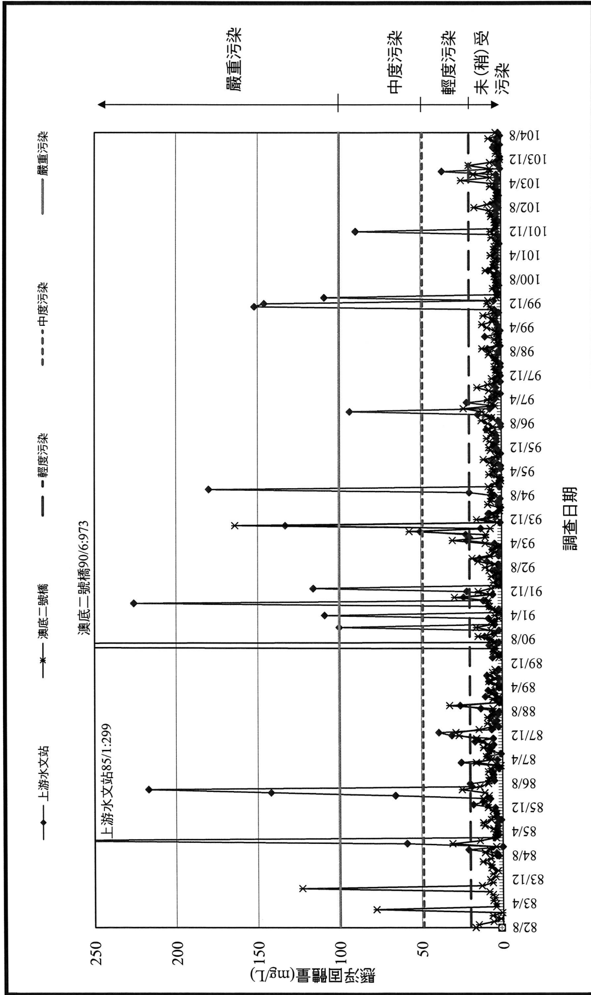
圖3.1-3 核四封存環境監測河川水質歷年調查懸浮固體濃度變化圖
