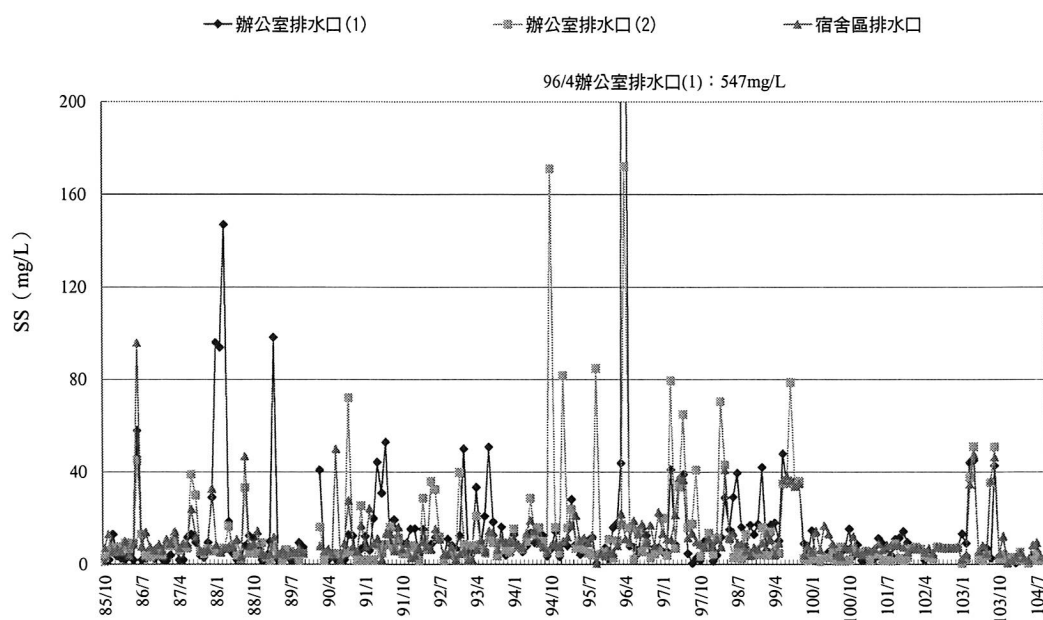
核四封存環境監測歷年廠區水質懸浮固體監測結果變化圖
