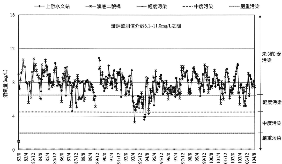
核四封存環境監測歷年河川水質之溶氧量監測結果變化圖
