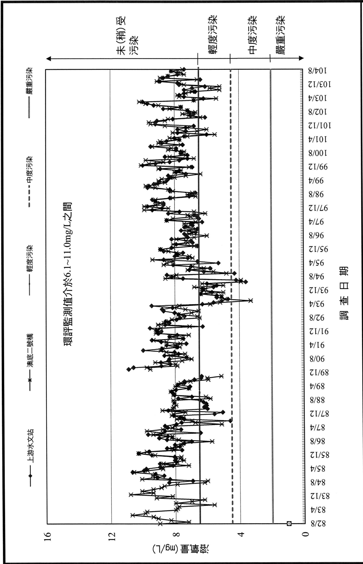
圖3.1-1 核四封存環境監測河川水質歷年調查溶氧量變化圖
