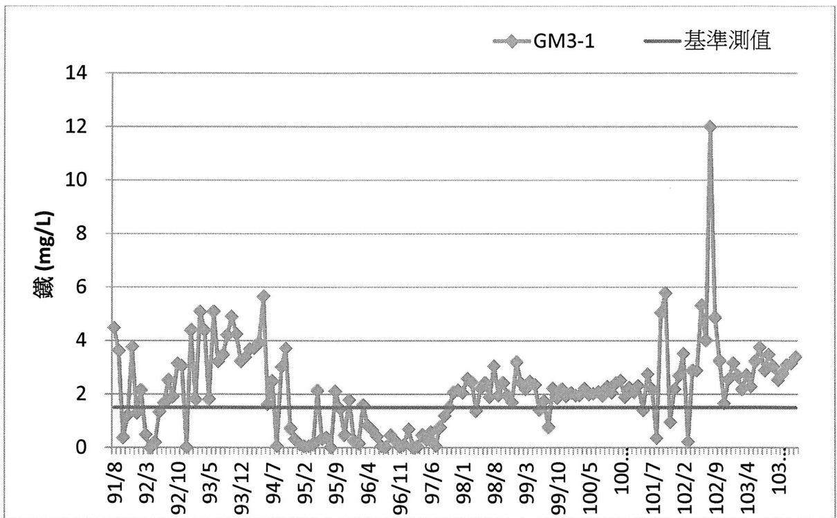
附圖 1 核四施工環境監測地下水 GM3-1 監測井鐵歷年監測趨勢圖
