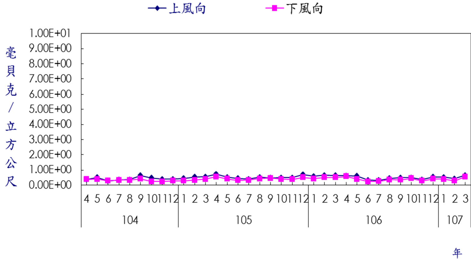
圖 15 核能三廠上下風向空氣微粒總貝他活度監測結果
