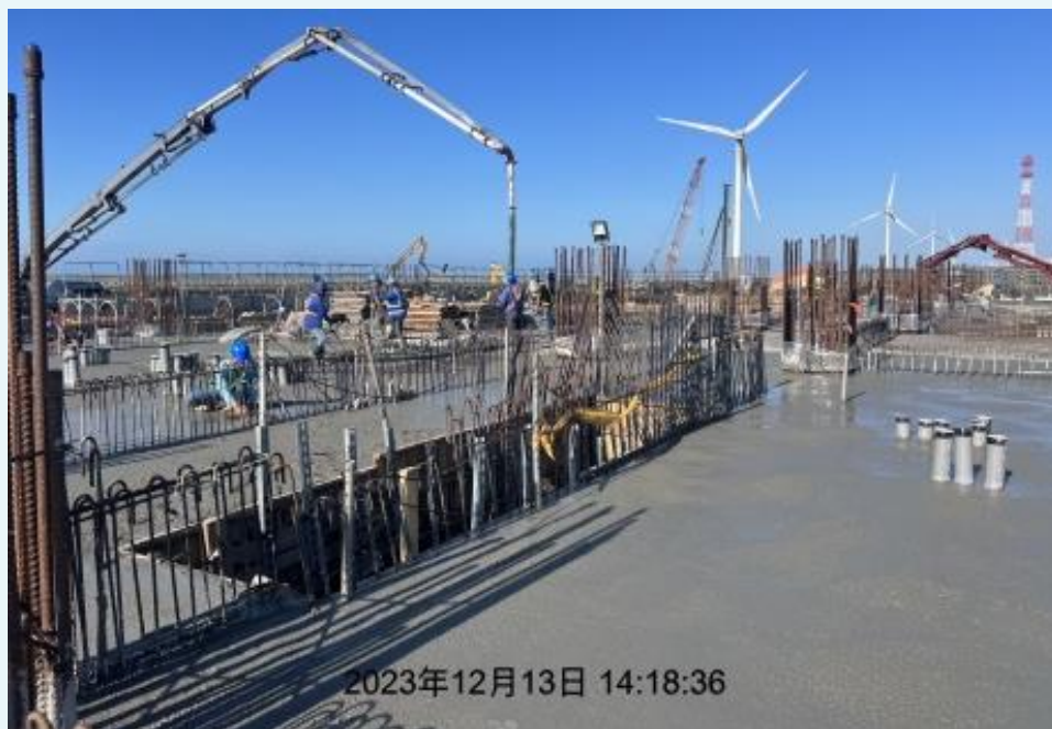
陸上電氣室1FL/B1F結構混凝土澆置施工抽查
