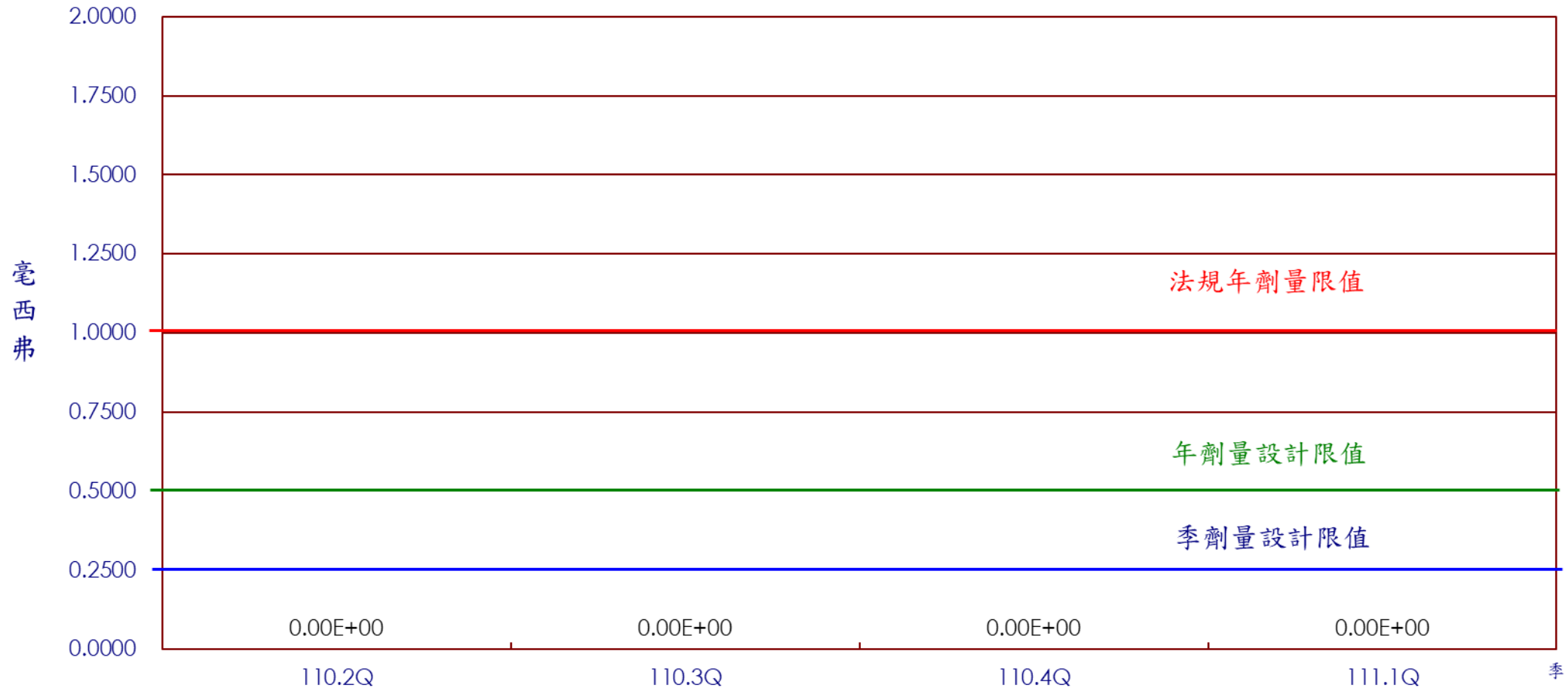
圖17 核能三廠111年第1季民眾最大個人全身劑量
