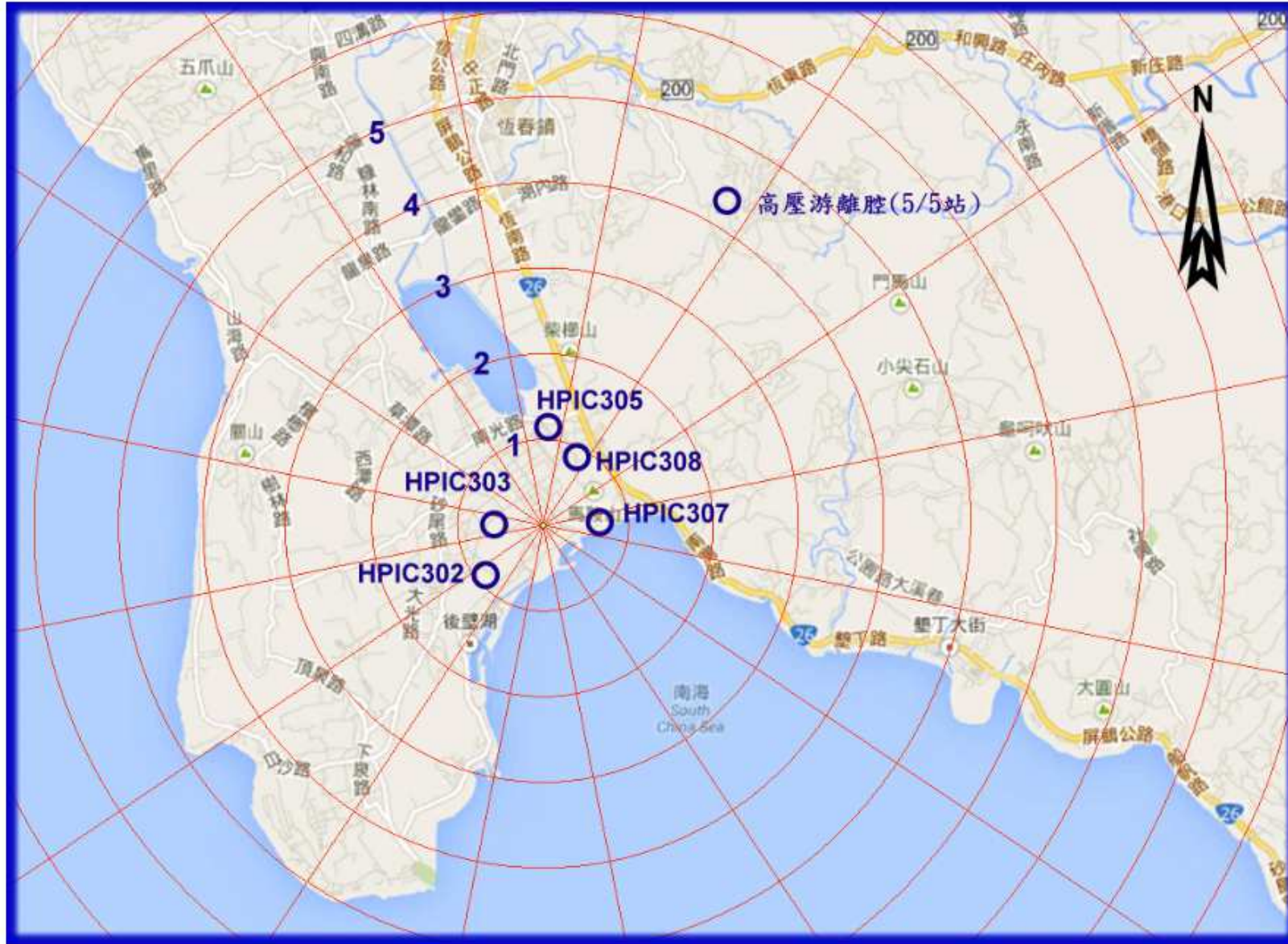
圖 3 核能三廠高壓游離腔監測站分佈圖
