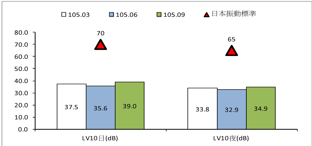
圖 2.2-2 計畫基地振動監測結果圖
