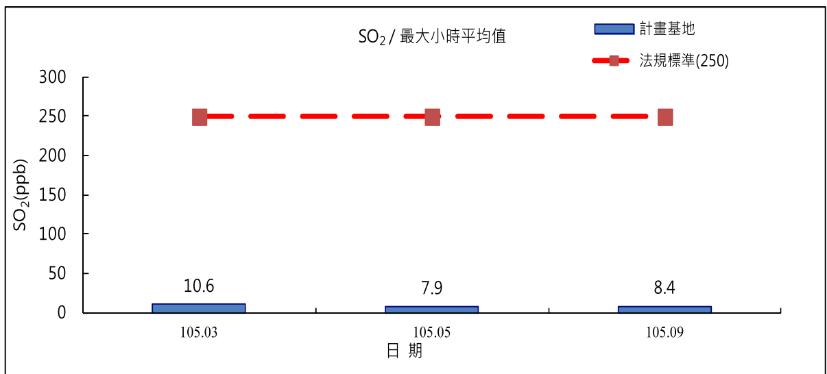
圖 2.1-1 空氣品質監測結果圖
