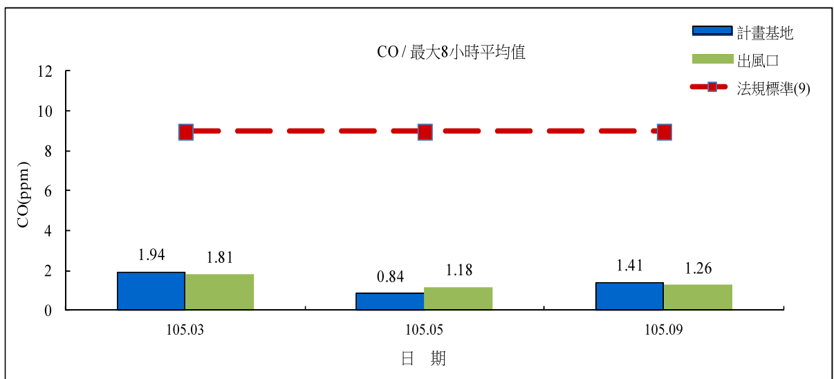
圖 2.1-1 空氣品質監測結果圖(續)
