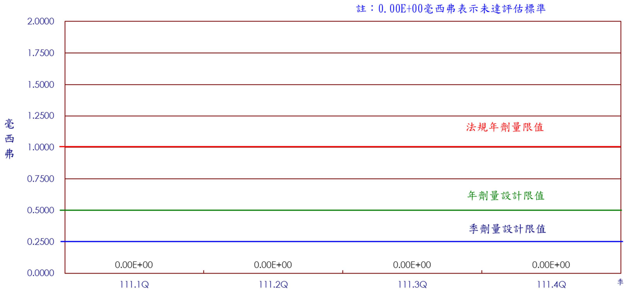
圖17 核能三廠111年第4季民眾最大個人全身劑量
