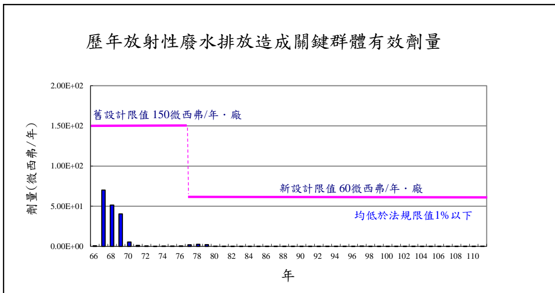
圖 15 歷年放射性廢水排放造成關鍵群體有效劑量趨勢
