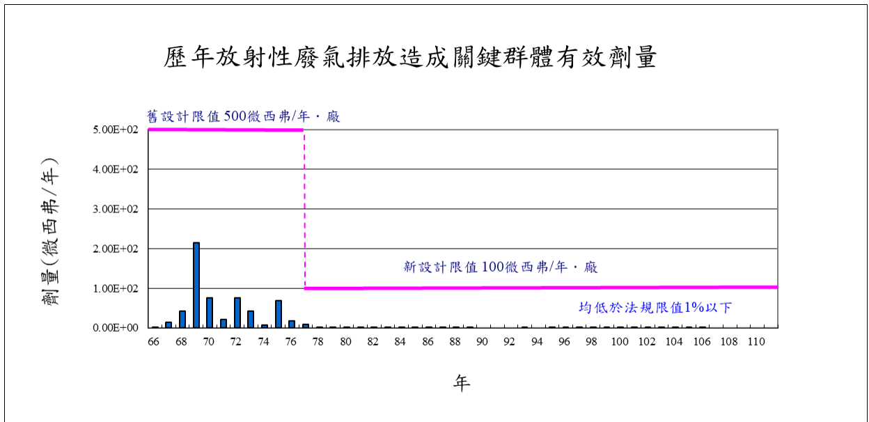
圖 14 歷年放射性廢氣排放造成關鍵群體有效劑量趨勢
