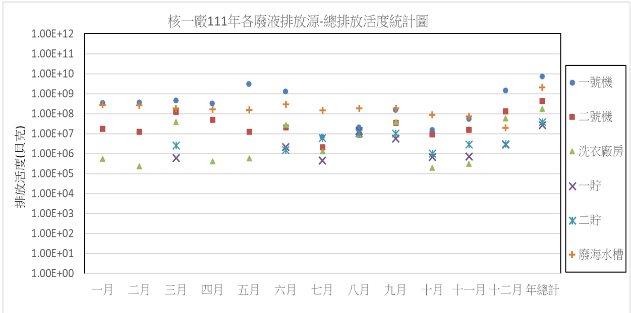
圖 12 111 年各廢水排放源總排放活度統計圖
