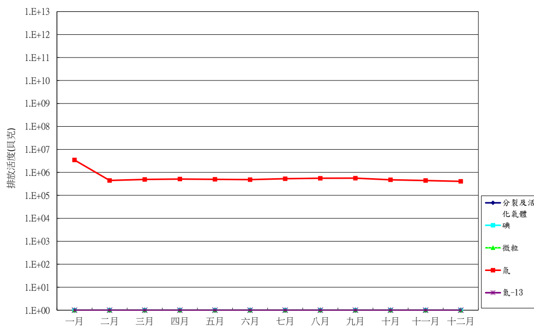
圖 7 111 年主煙囪放射性廢氣排放活度統計圖
