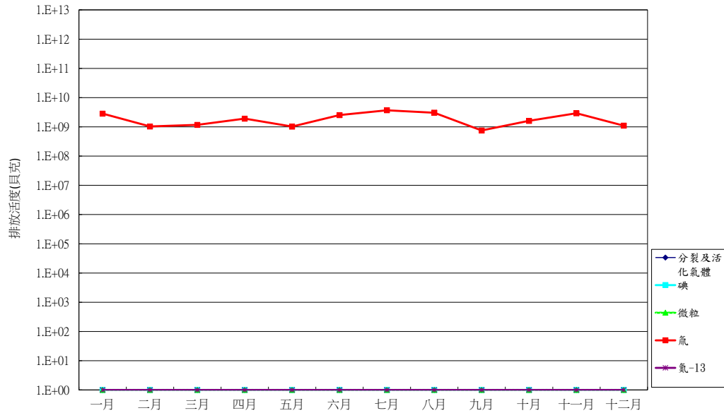
圖 5 111 年一號機放射性廢氣排放活度統計圖
