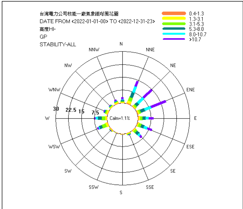
核一廠高塔氣象風花圖
