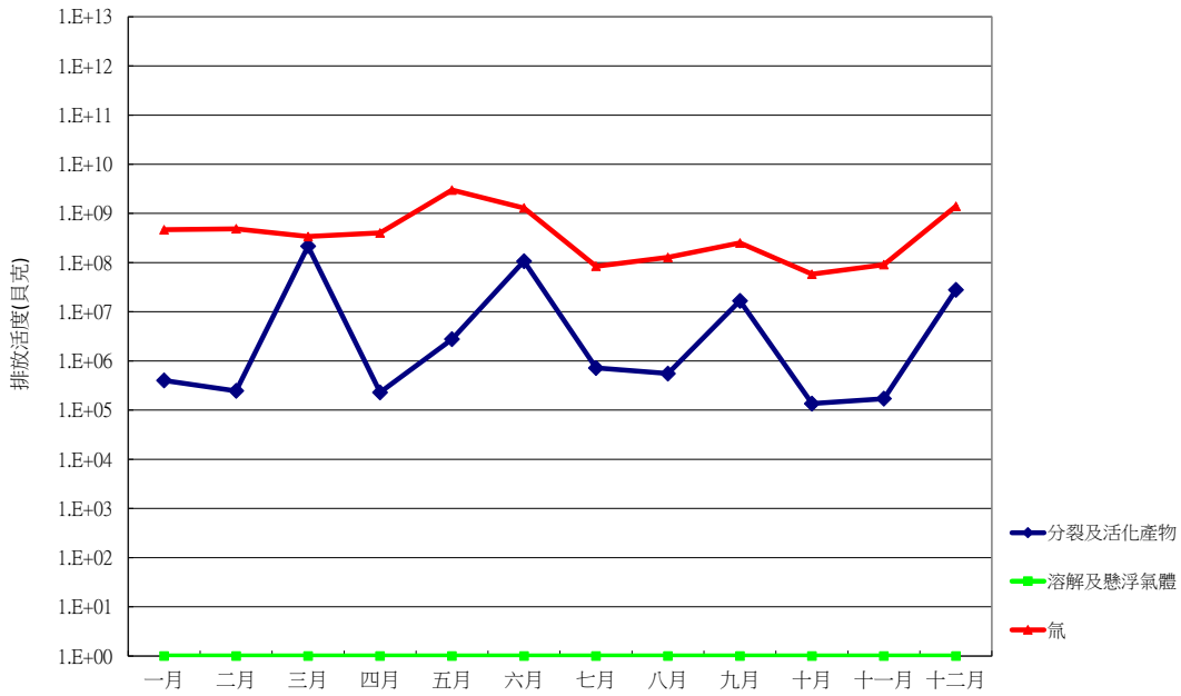
圖 10 111 年一號機放射性廢水排放活度統計圖
