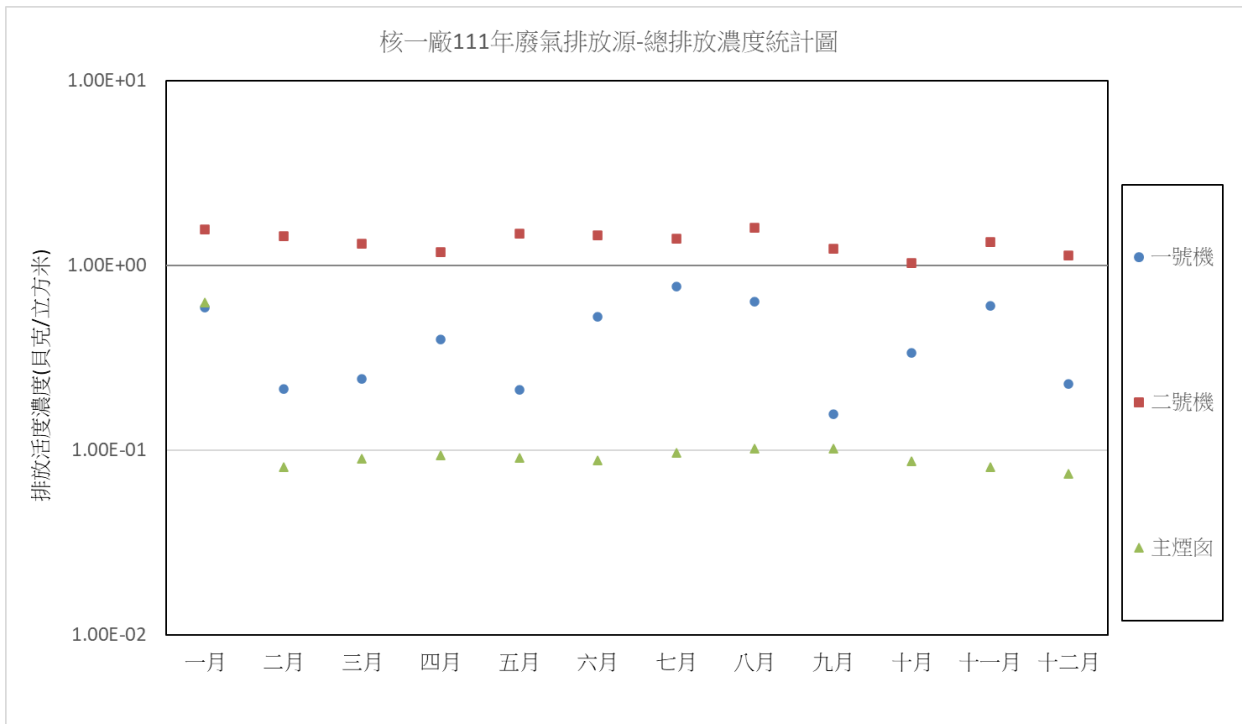
圖 9 111 年各廢氣排放源總排放濃度統計圖
