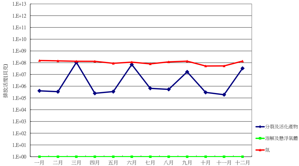
圖 11 111 年二號機放射性廢水排放活度統計圖
