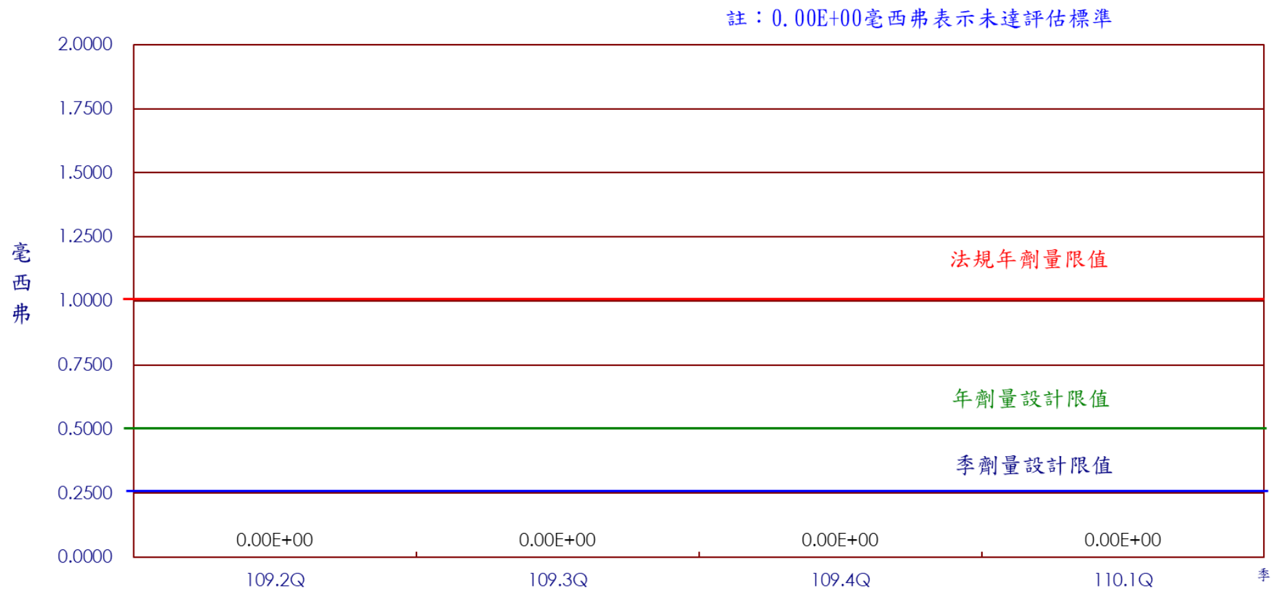
圖17 核能三廠110年第1季民眾最大個人全身劑量
