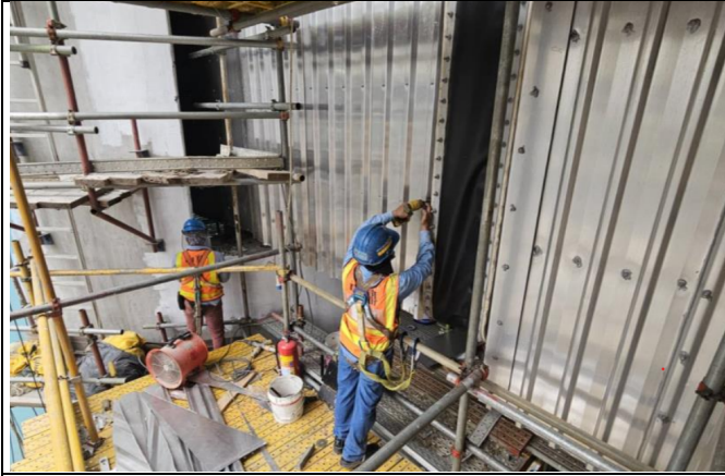
主發電設備工程 Unit 2 HRSG 2-2 設備安裝
