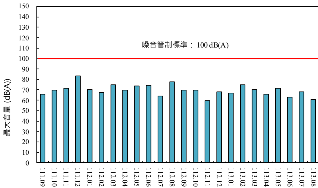
圖 3.1.1-1 歷次營建噪音均能音量值及最大音量值變化圖
