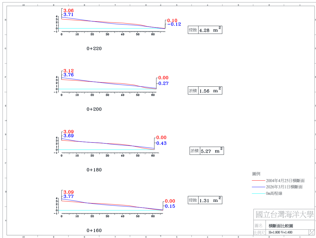
圖 4-4(h) 2026 年 03 月 01 日 A 監測區橫斷面比較圖
