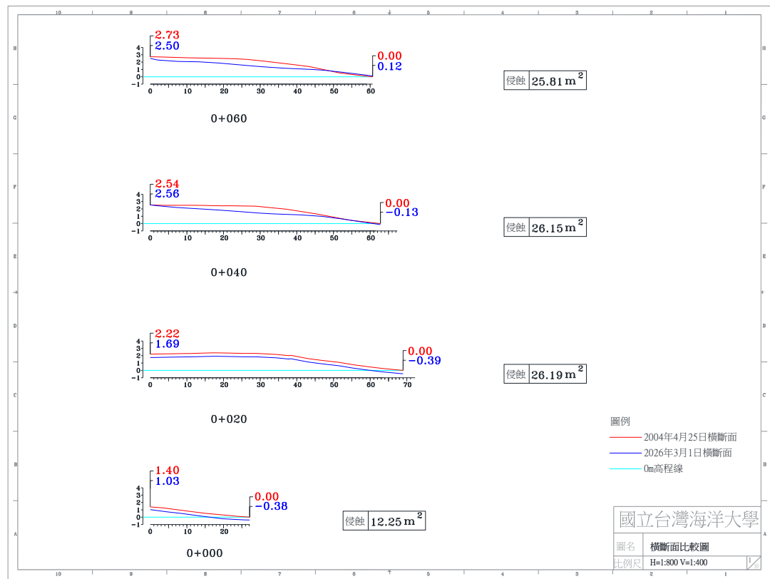
圖 4-4(j) 2026 年 03 月 01 日 A 監測區橫斷面比較圖
