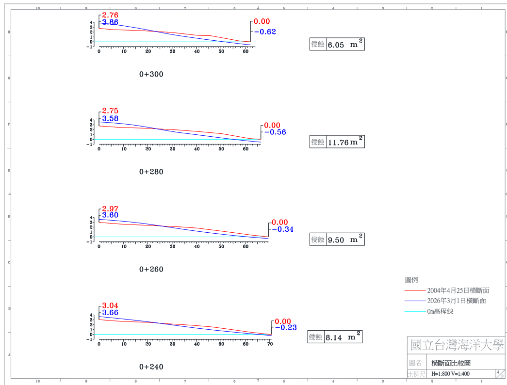
圖 4-4(g) 2026 年 03 月 01 日 A 監測區橫斷面比較圖
