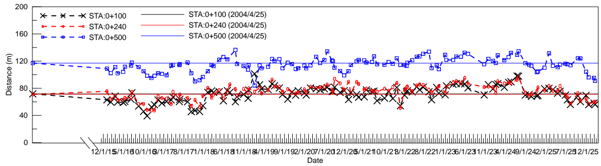
圖 4-21 岸線斷面沙灘寬度變化圖(2026/03/01)
