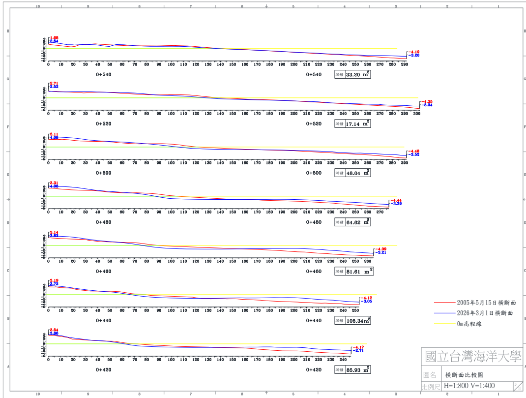
圖 4-5(c) 2026 年 03 月 01 日 B 監測區橫斷面比較圖
