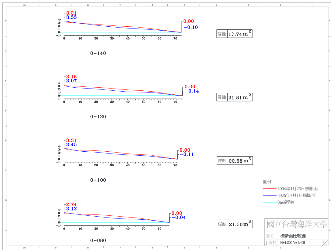
圖 4-4(i) 2026 年 03 月 01 日 A 監測區橫斷面比較圖
