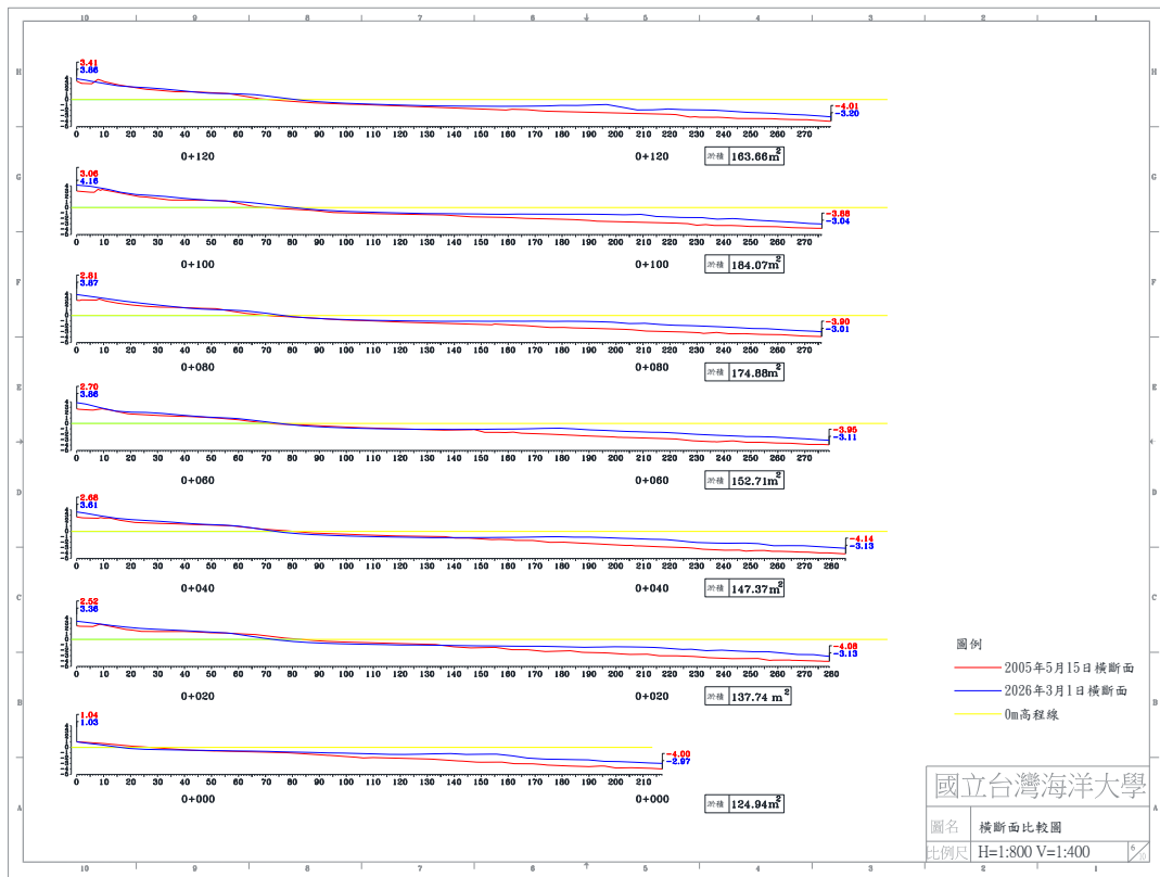
圖 4-5(f) 2026 年 03 月 01 日 B 監測區橫断面比較圖
