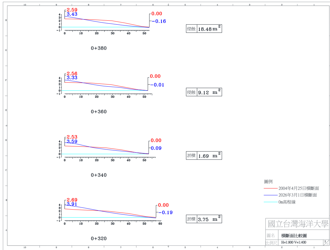
圖 4-4(f) 2026 年 03 月 01 日 A 監測區橫斷面比較圖
