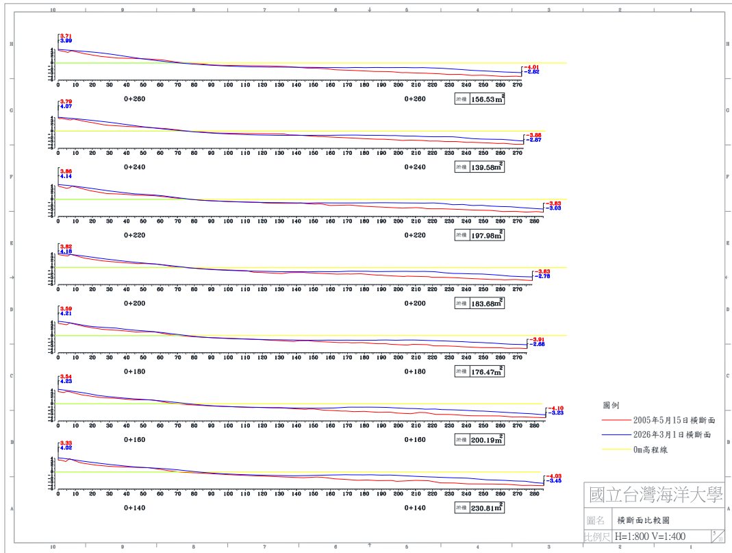
圖 4-5(e) 2026 年 03 月 01 日 B 監測區橫断面比較圖
