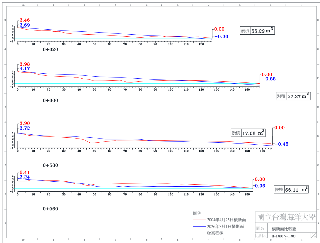
圖 4-4(c) 2026 年 03 月 01 日 A 監測區橫斷面比較圖
