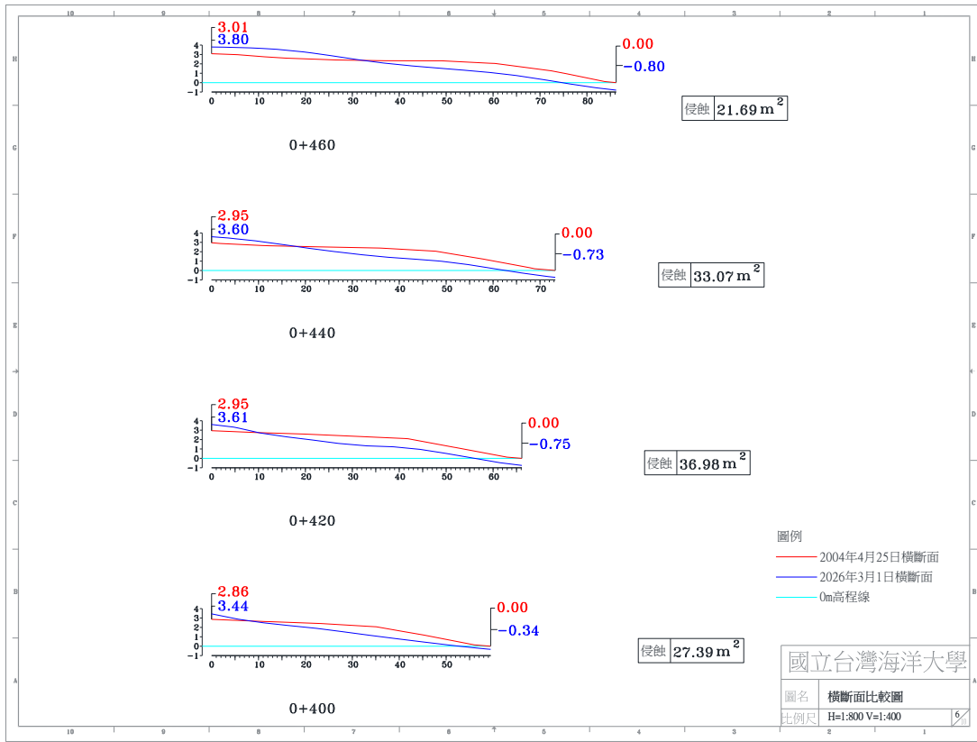
圖 4-4(e) 2026 年 03 月 01 日 A 監測區橫斷面比較圖
