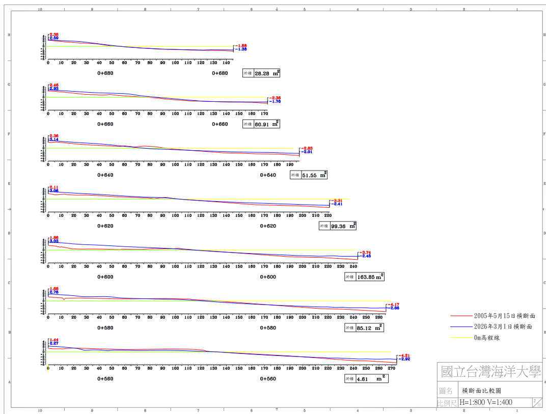
圖 4-5(b) 2026 年 03 月 01 日 B 監測區橫斷面比較圖
