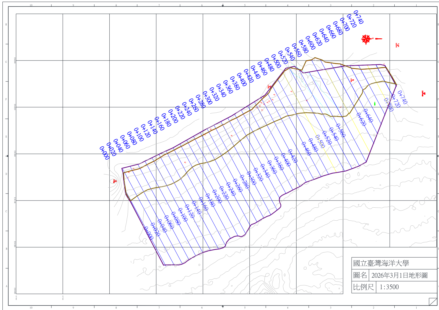
圖 4-1 2026 年 3 月 1 日監測地形
