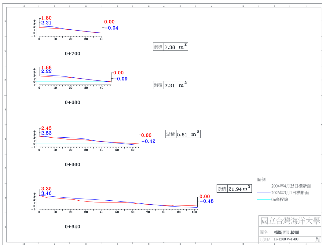
圖 4-4(b) 2026 年 03 月 01 日 A 監測區橫斷面比較圖
