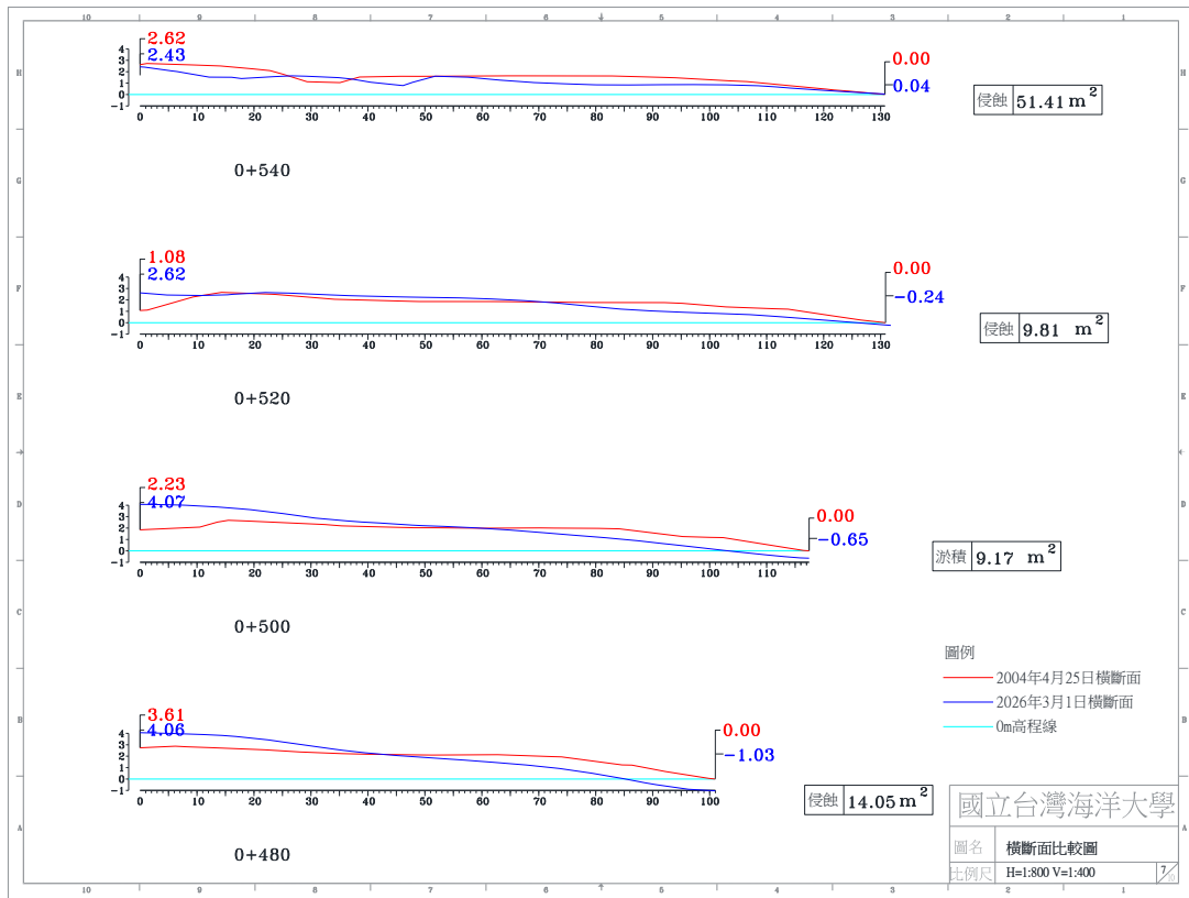
圖 4-4(d) 2026 年 03 月 01 日 A 監測區橫斷面比較圖
