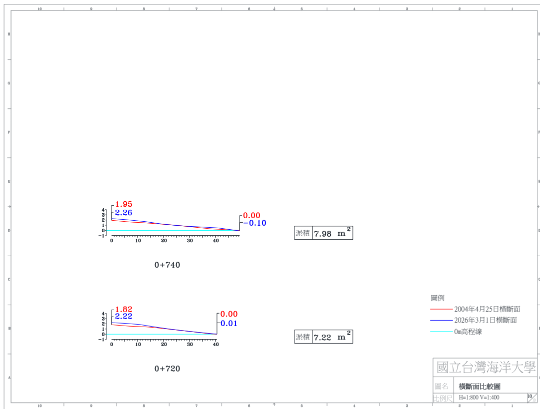
圖 4-4(a) 2026 年 03 月 01 日 A 監測區橫斷面比較圖
