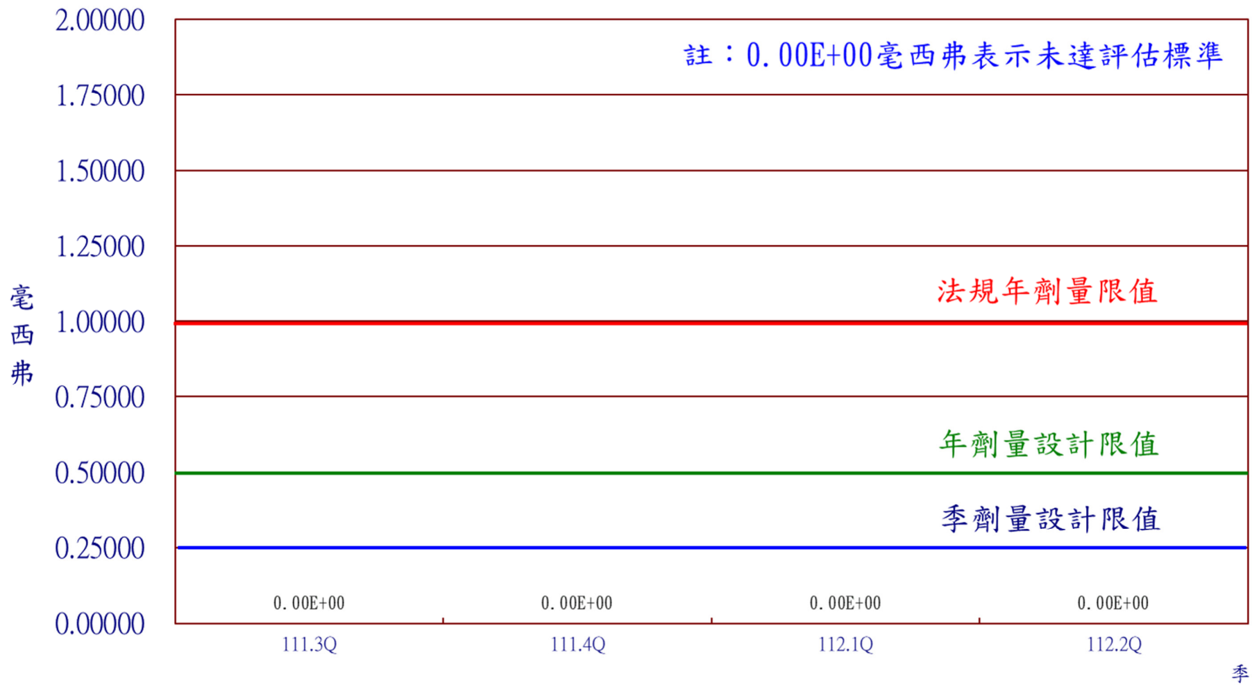
圖18 核能一廠112年第2季民眾最大個人全身劑量
