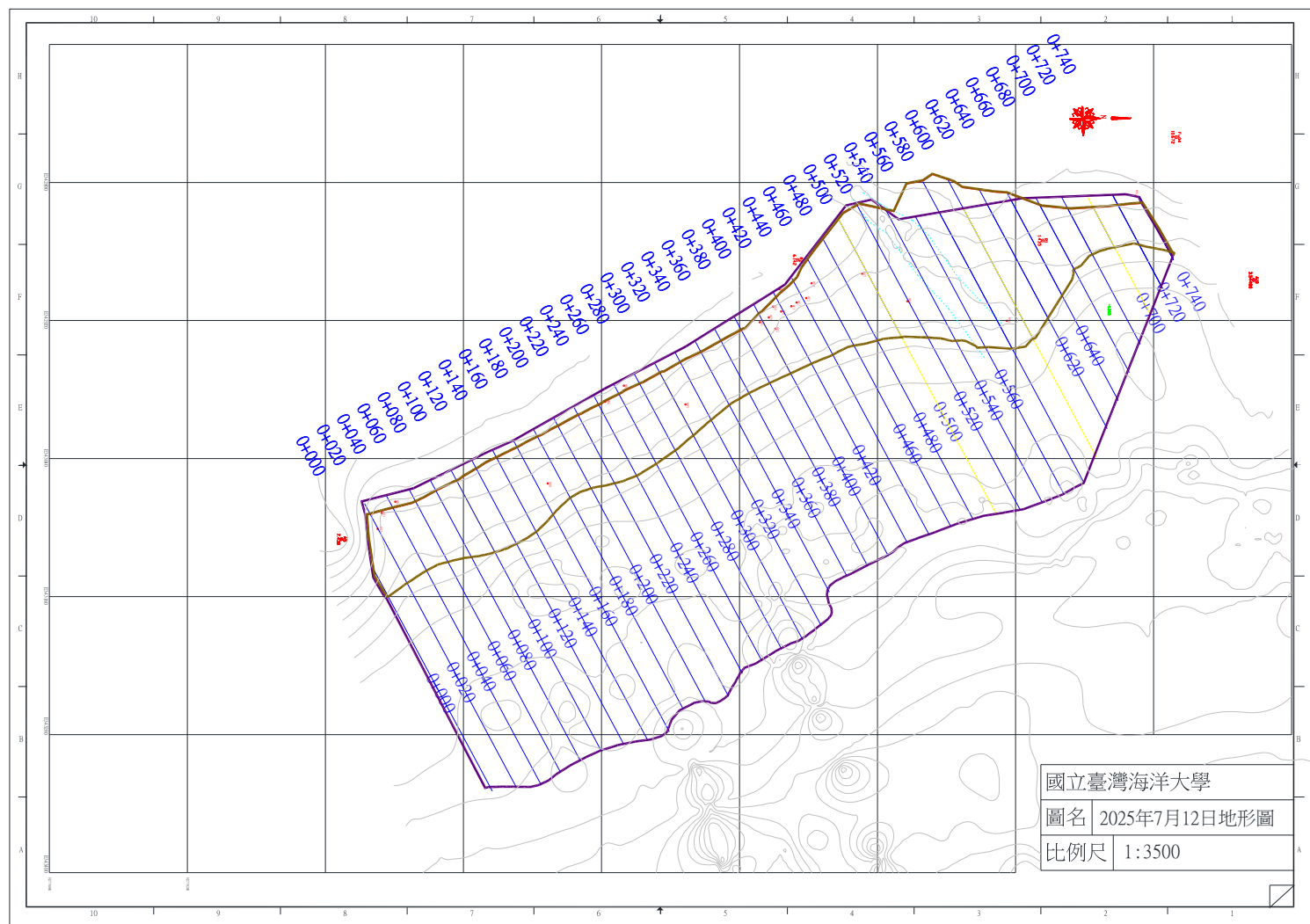
圖 4-1 2025 年 7 月 12 日監測地形
