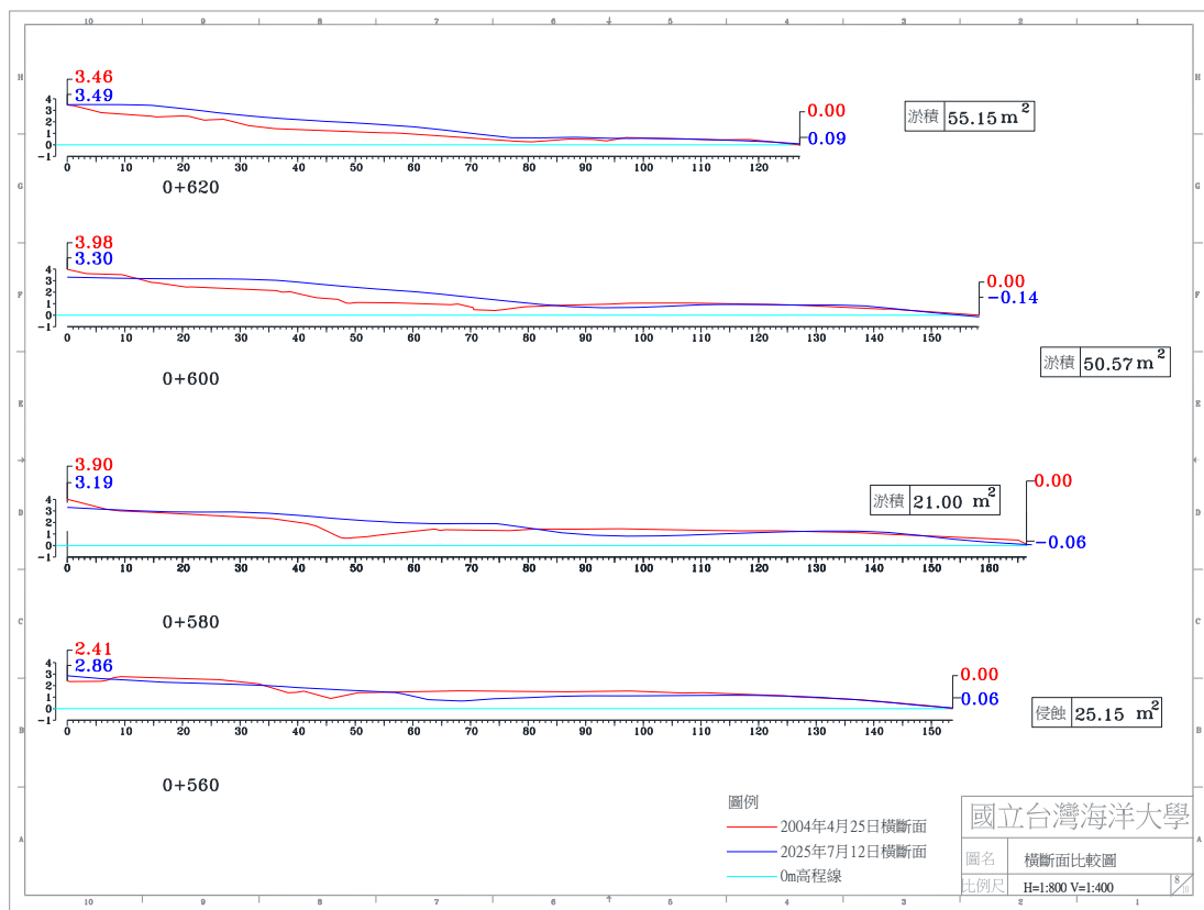
圖 4-4(c) 2025 年 7 月 12 日 A 監測區橫斷面比較圖
