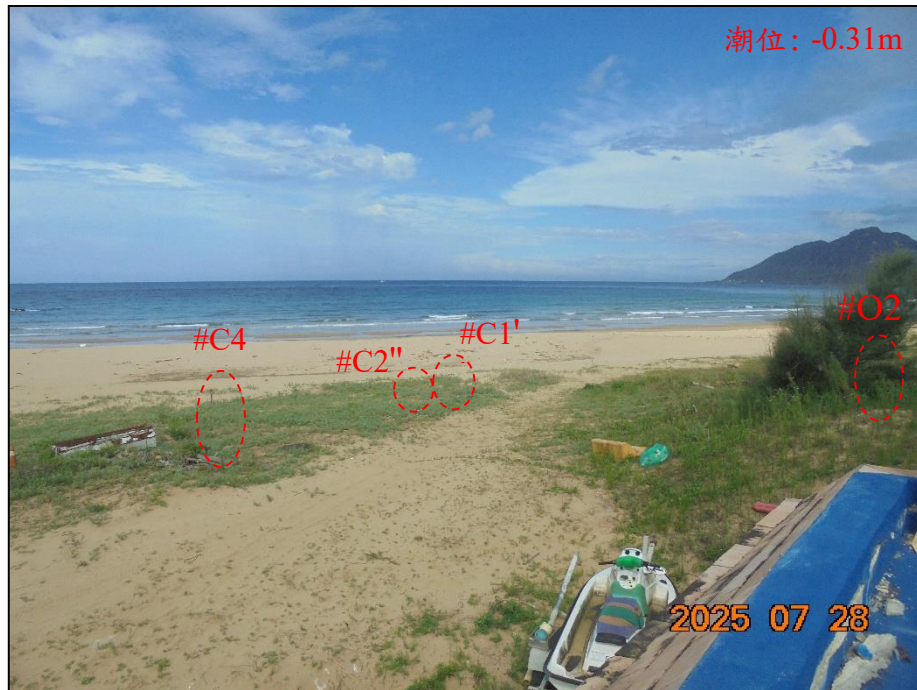
圖 3-12 小舞台南側輔助觀測樁位置圖（2025/07/28）
