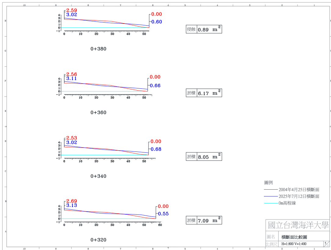
圖 4-4(f) 2025 年 7 月 12 日 A 監測區橫斷面比較圖
