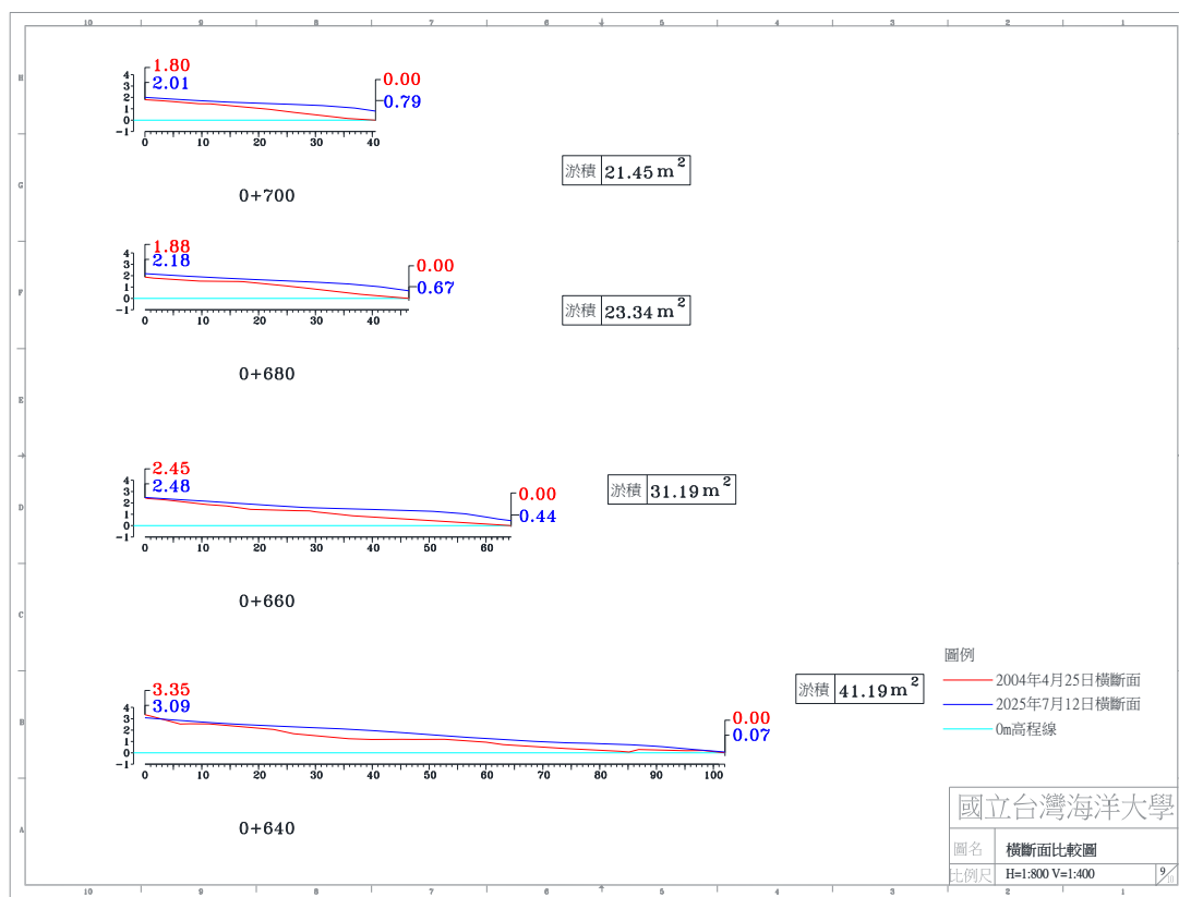
圖 4-4(b) 2025 年 7 月 12 日 A 監測區橫斷面比較圖
