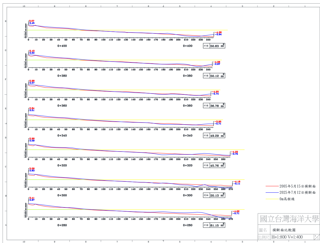
圖 4-5(d) 2025 年 7 月 12 日 B 監測區橫斷面比較圖
