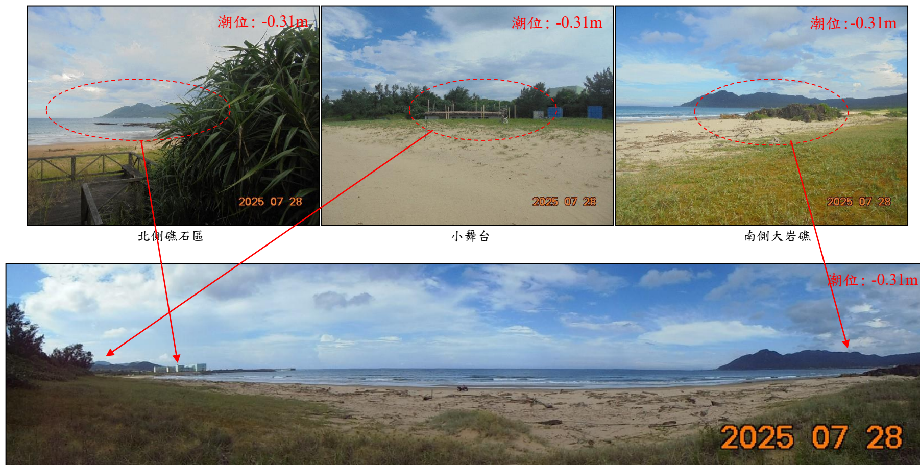
圖 3-8 鹽寮海岸短期性養灘區地形地貌圖 (2025/07/28)
