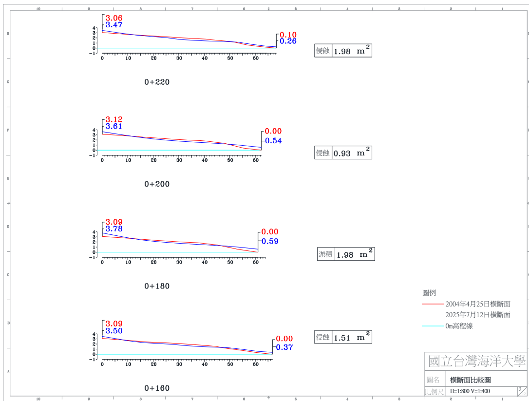
圖 4-4(h) 2025 年 7 月 12 日 A 監測區橫斷面比較圖
