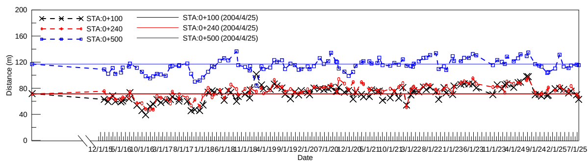
圖 4-21 岸線斷面沙灘寬度變化圖(2025/07/12)
