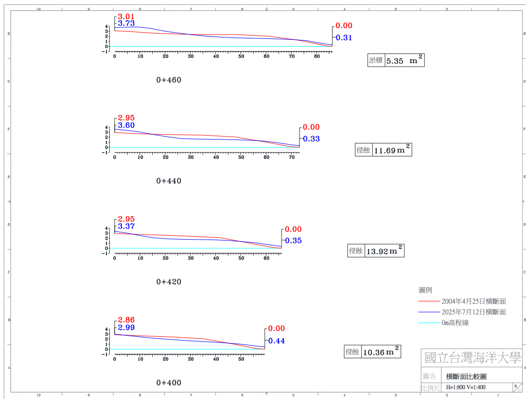
圖 4-4(e) 2025 年 7 月 12 日 A 監測區橫斷面比較圖
