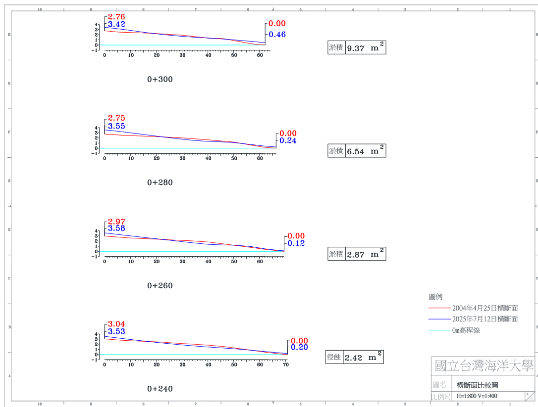
圖 4-4(g) 2025 年 7 月 12 日 A 監測區橫斷面比較圖
