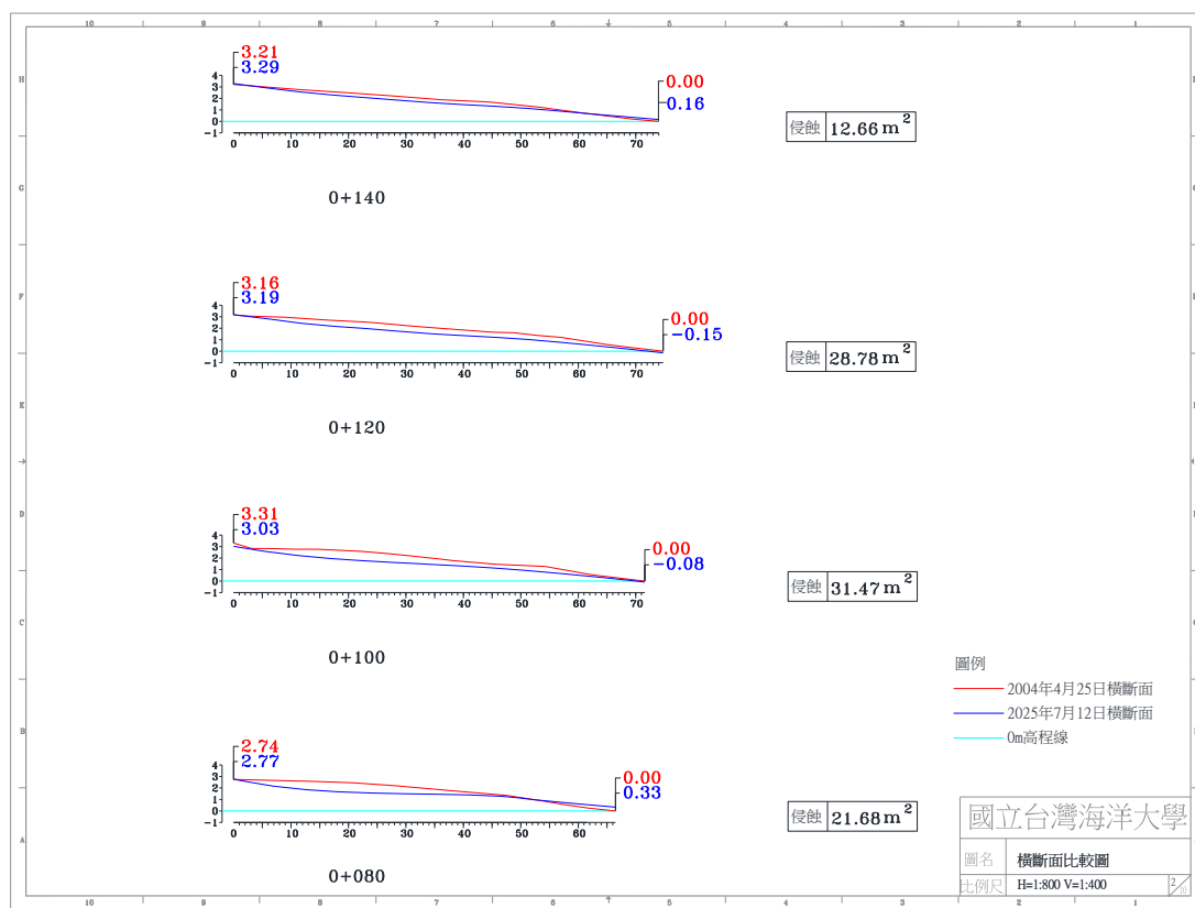
圖 4-4(i) 2025 年 7 月 12 日 A 監測區橫斷面比較圖
