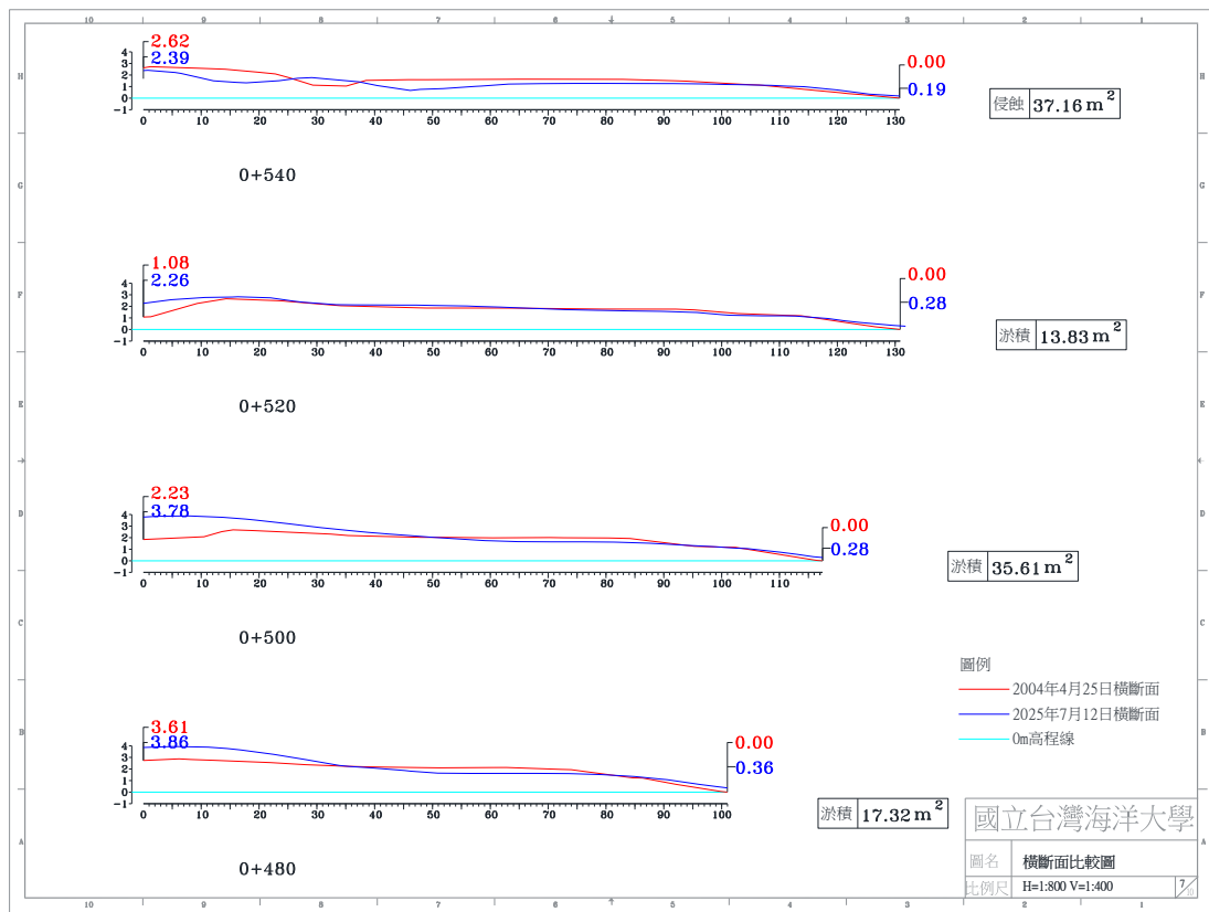
圖 4-4(d) 2025 年 7 月 12 日 A 監測區橫斷面比較圖
