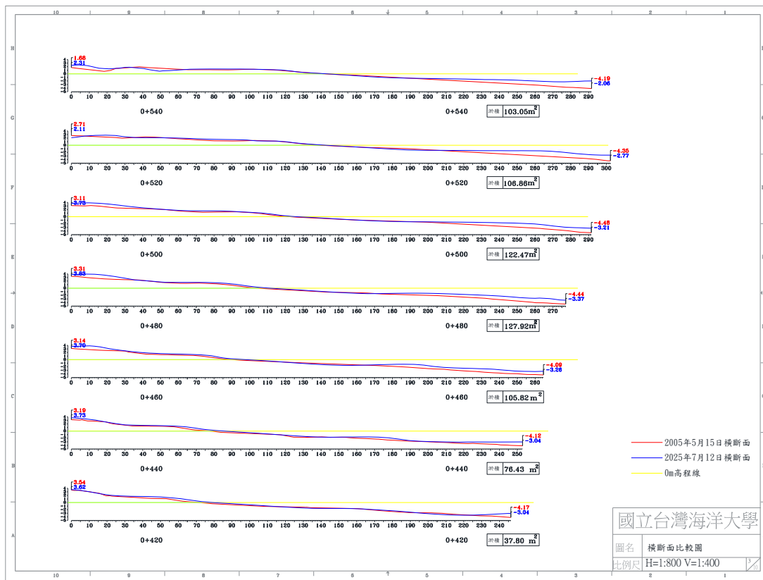
圖 4-5(c) 2025 年 7 月 12 日 B 監測區橫斷面比較圖
