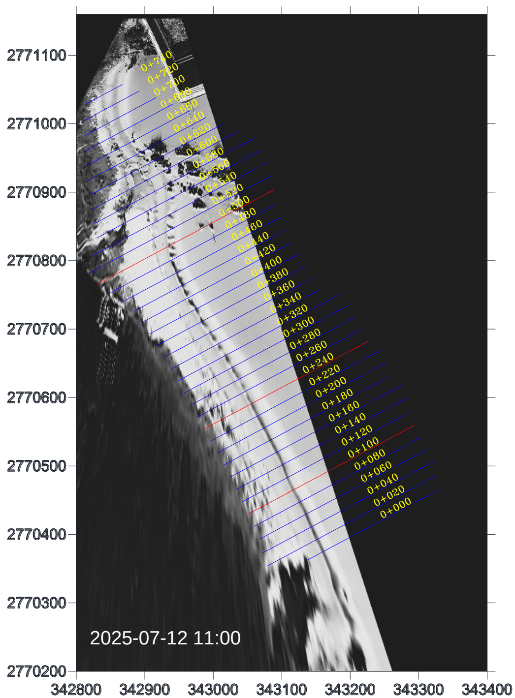
圖 4-19 鹽寮海岸地形影像全景圖(2025/07/12 11:00)
