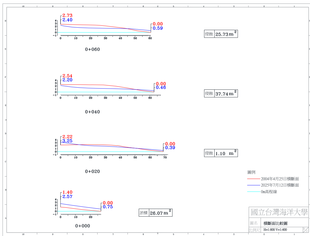
圖 4-4(j) 2025 年 7 月 12 日 A 監測區橫斷面比較圖
