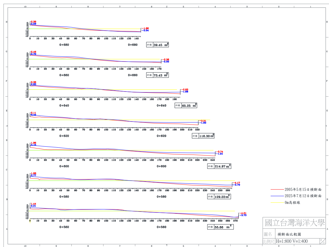
圖 4-5(b) 2025 年 7 月 12 日 B 監測區橫斷面比較圖
