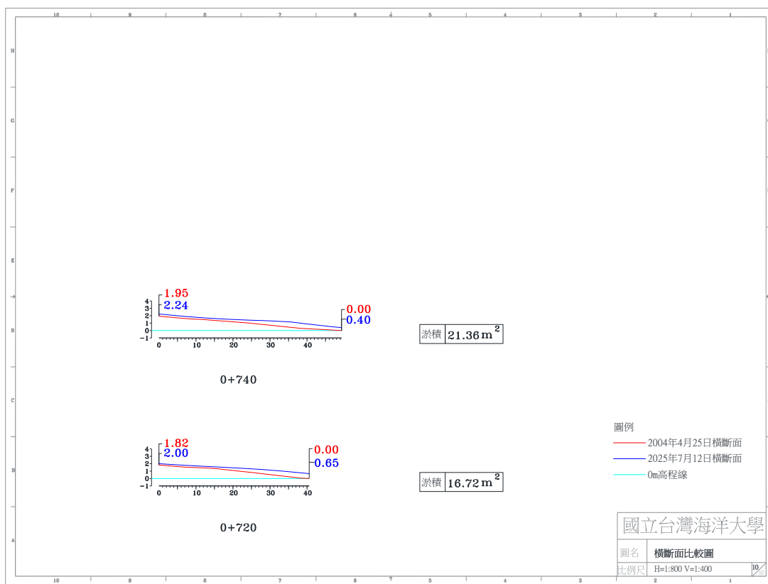
圖 4-4(a) 2025 年 7 月 12 日 A 監測區橫斷面比較圖
