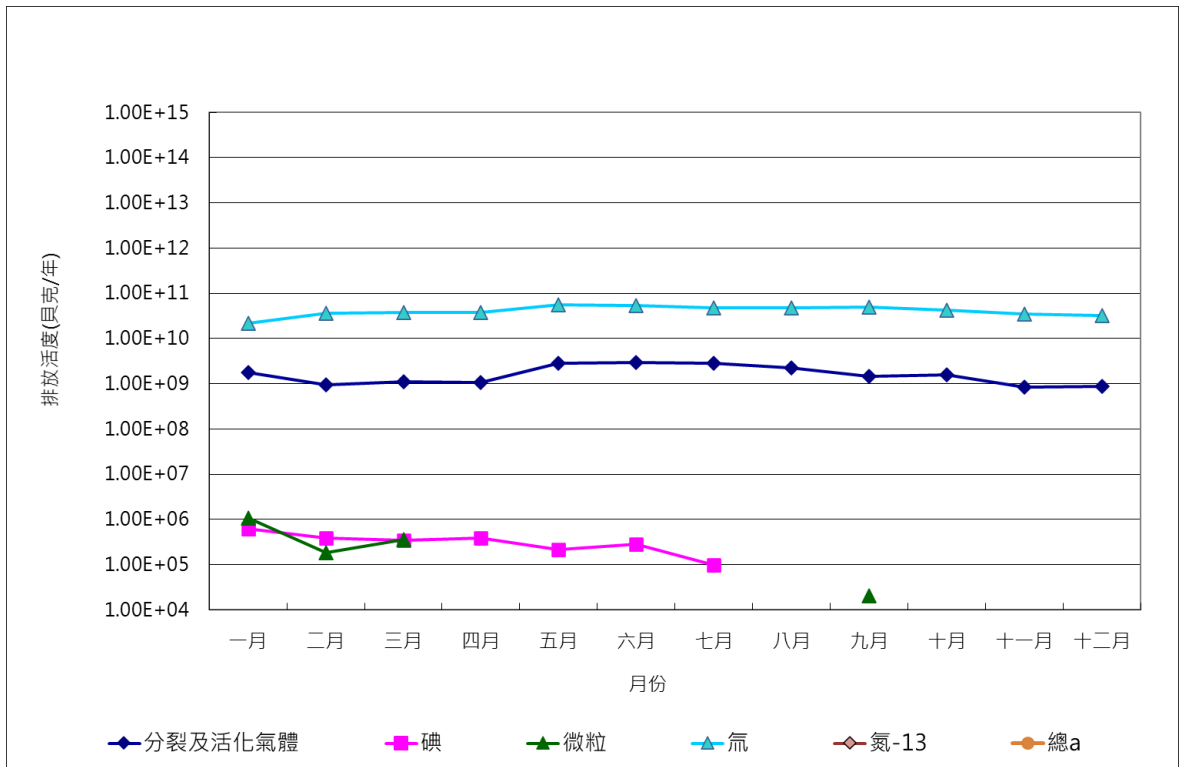
圖 9 110 年 2 號機放射性廢氣排放活度統計圖
