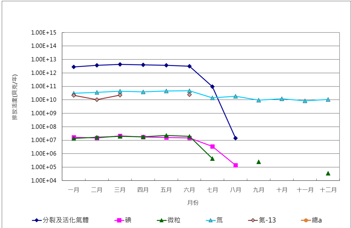
圖 8 110 年 1 號機放射性廢氣排放活度統計圖
