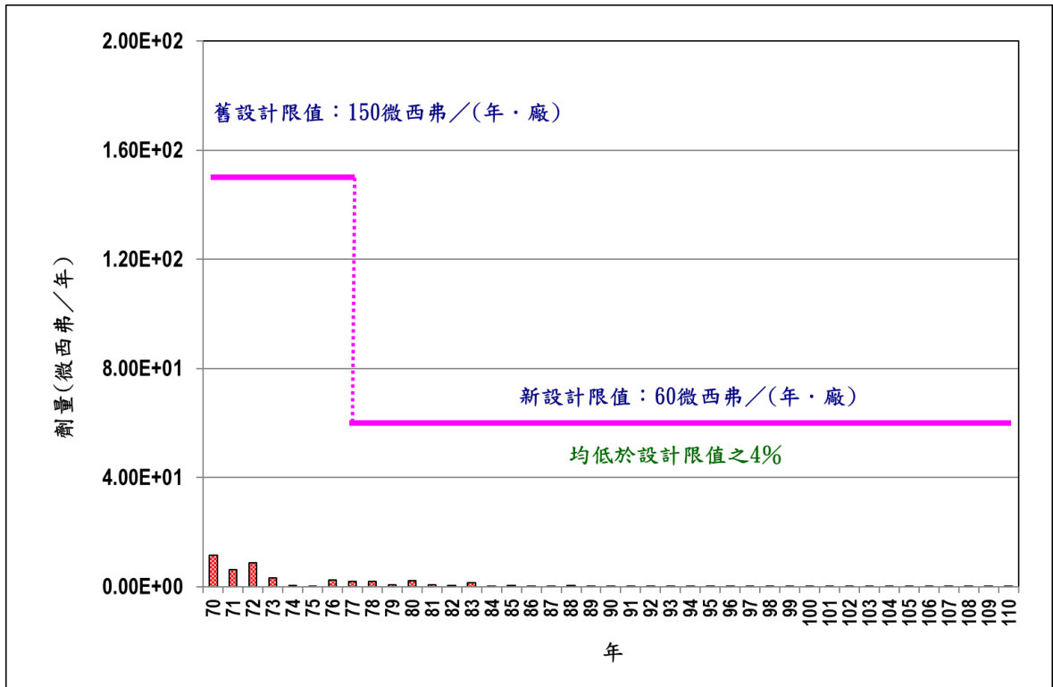
圖 12 歷年放射性廢水排放造成關鍵群體有效劑量趨勢圖
