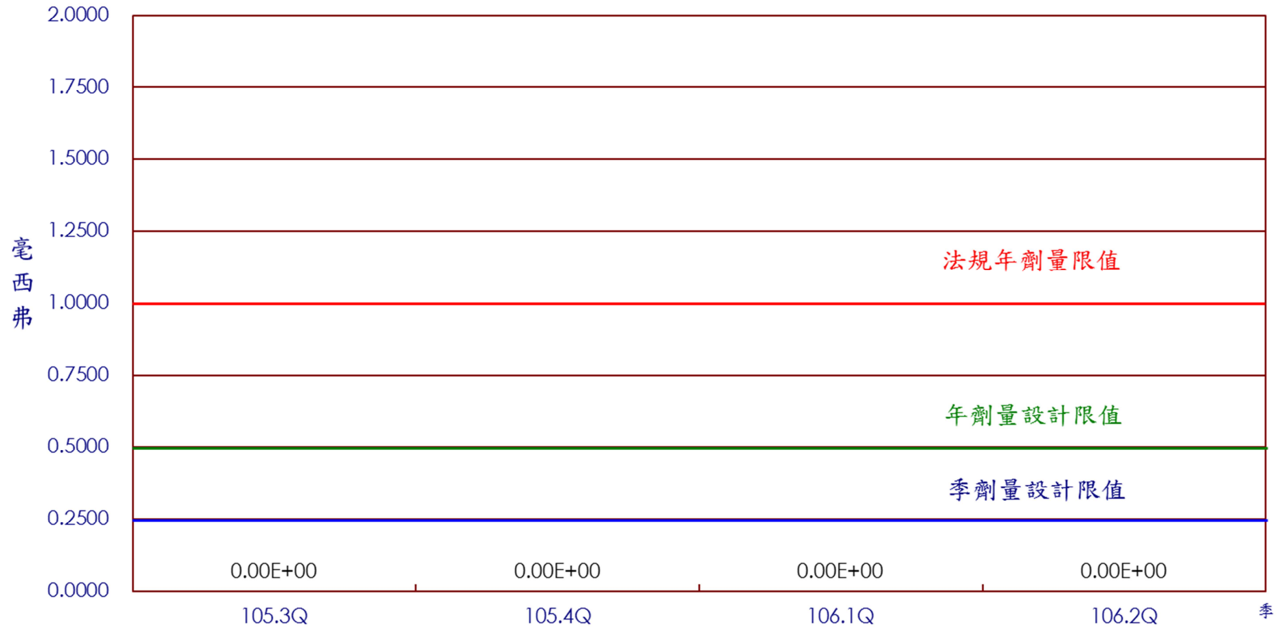
圖17 核能三廠106年第2季民眾最大個人全身劑量
