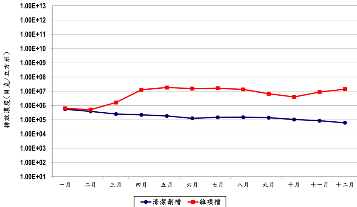
圖十 核二廠113年各廢液排放源-總排放濃度統計圖
