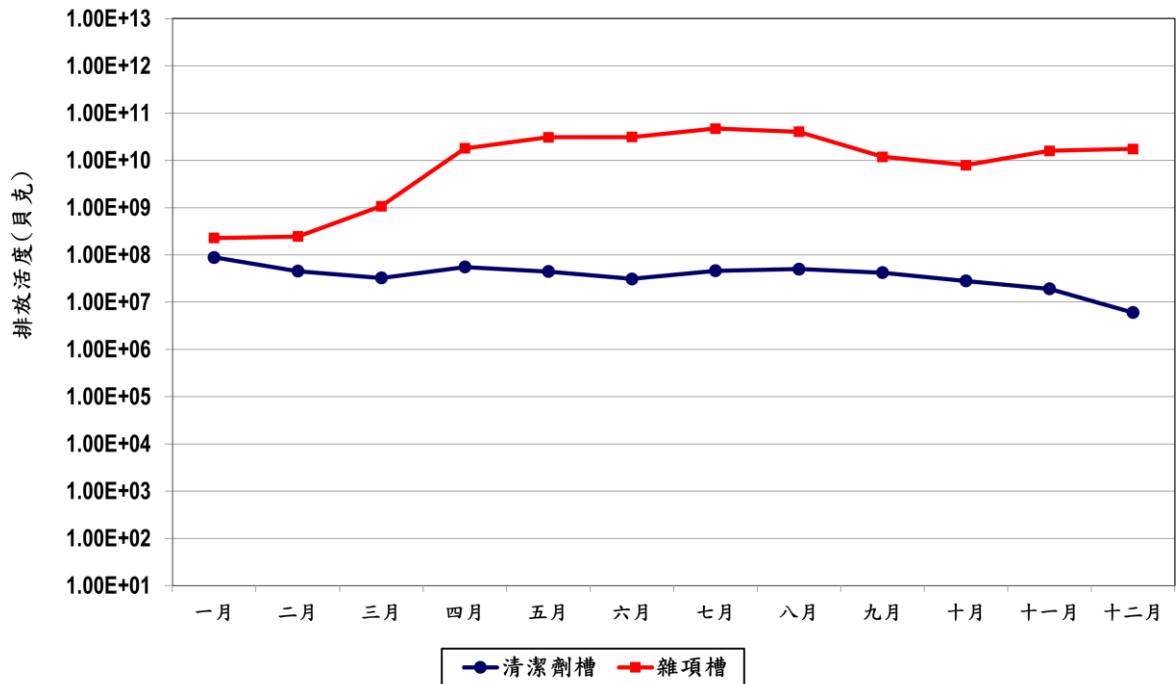
圖九 核二廠113年各廢液排放源-總排放活度統計圖
