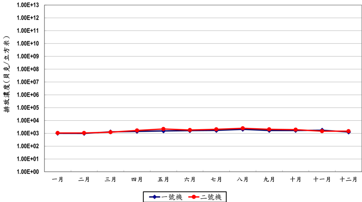
圖七 核二廠113年廢氣排放源-總排放濃度統計圖
