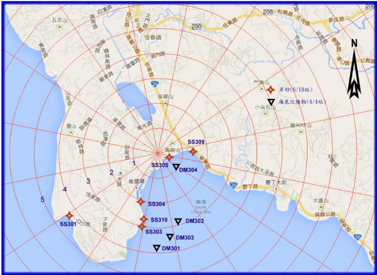
圖 10 核能三廠岸砂取樣站分佈圖(5 公里內)
